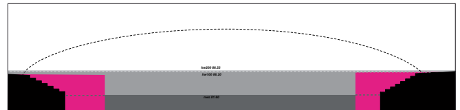
Abb.2 Rückbau (pink) der Molenköpfe (Schnitt)
