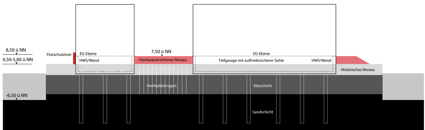
Prinzipischnitt Warftenkonzept Dalmannkai
