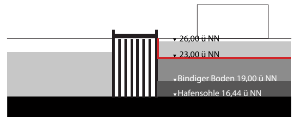
Längsschnitt Holzhafen-Innenhafen
